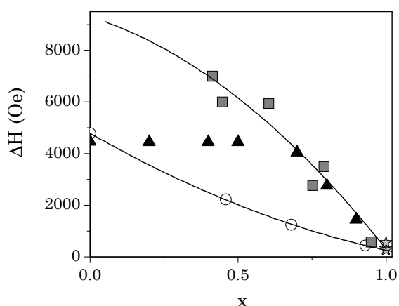
Рис.1 - Ширина линии ферромагнитного резонанса в порошках композиционных частиц в зависимости от весовой доли немагнитной фазы (x). Пустые кружки – CoNiP@NiP, серые квадраты – CoFeP@NiP, черные треугольники - CoP@Cu. Серыми звездочками показаны опорные величины ширины линии, измеренные на покрытиях состава аналогичного составу магнитных частиц
